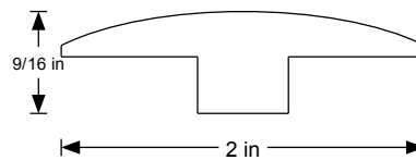
9/16" T-MOLDING
